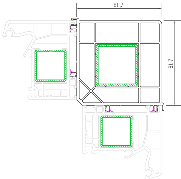
accouplement 90°
