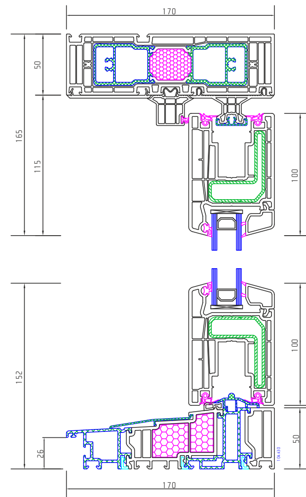
Coupe verticale
