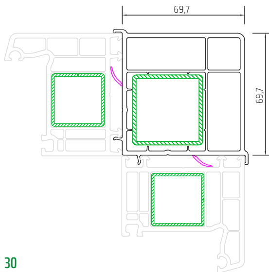
accouplement 90'
