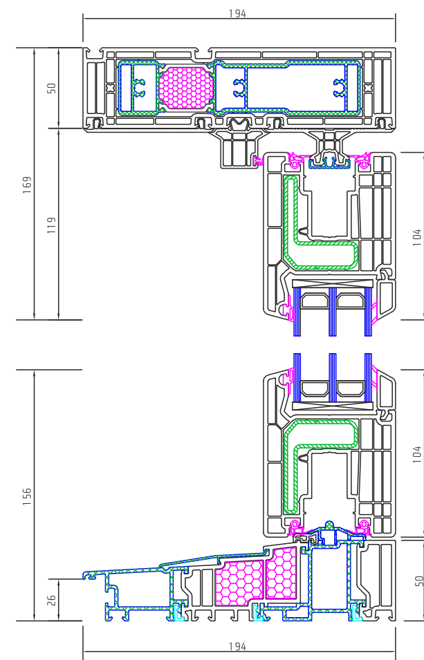
Coupe verticale
