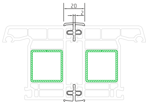
accouplement 90'
