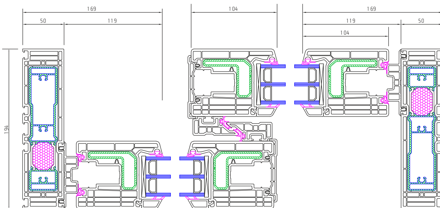
Coupe transversale
