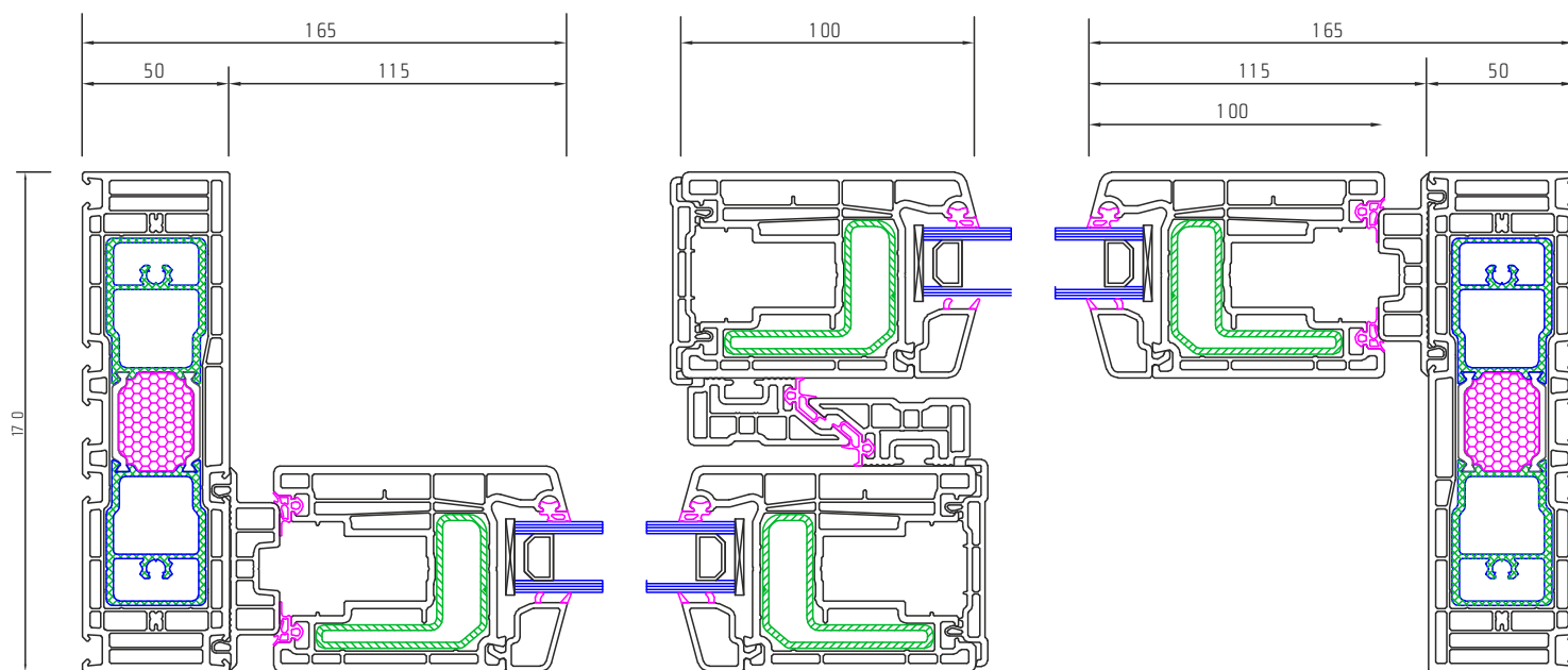
Coupe transversale
